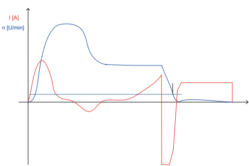
使用先行停止识别功能旋盖时的转速和电流（扭矩）趋势图
